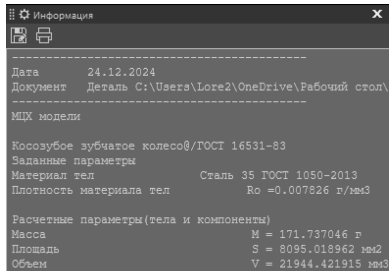
Рисунок 15 – МЦХ модели
